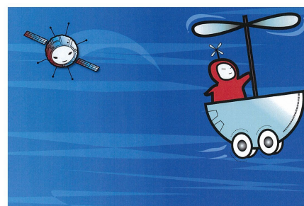
3 運動エネルギー&ポロニウム
