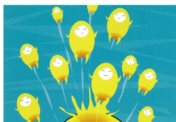
5 ニュートリノ
